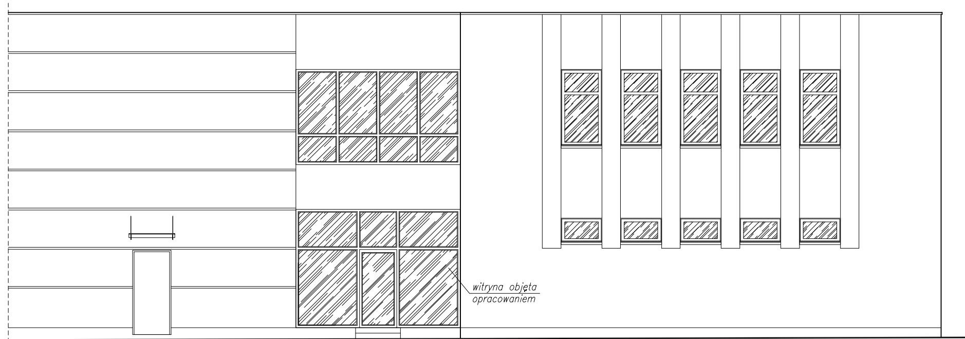
elevacja południowa
